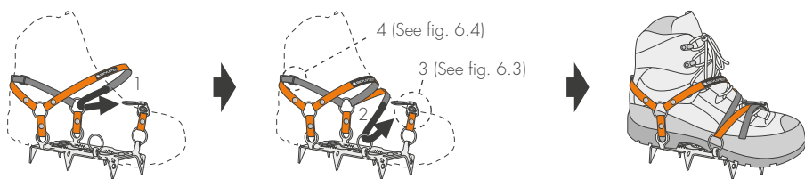
5.1 - MINI CRAMPON 6P
