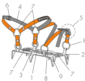
3.1 - MINI CRAMPON 6P
